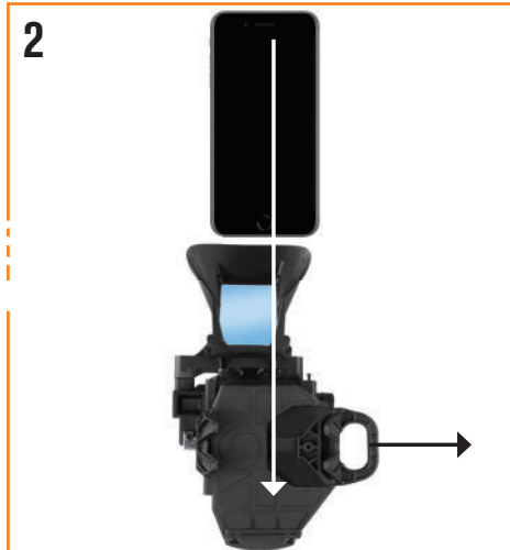
2. Legen Sie Ihr Smartphone dann in das StarSense-Dock.
